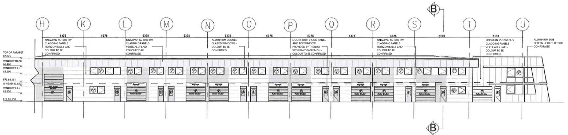
Elevation A-A
