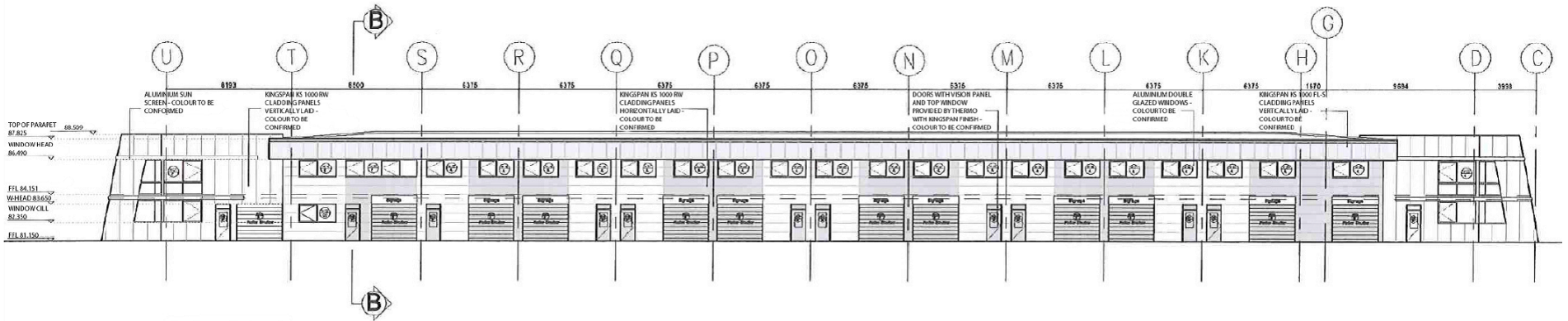
Elevation C-C
