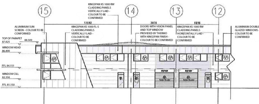
Elevation D-D
