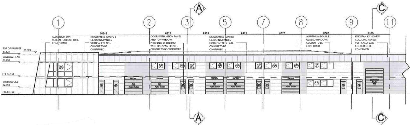
Elevation G-G
