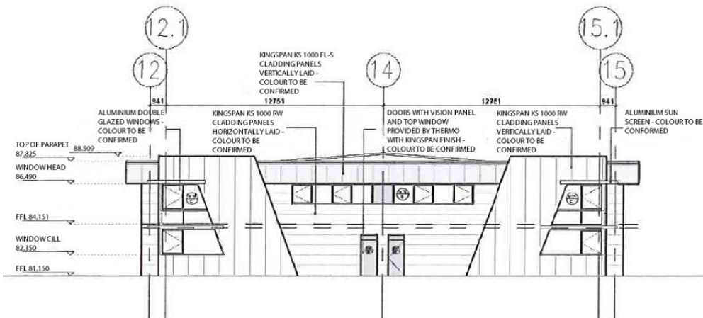
Elevation B-B
